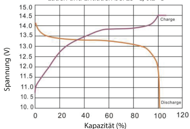
Laden und Entladen bei 25 °C, 0.2 °C
