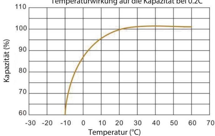
Temperaturwirkung auf die Kapazität bei 0.2C
