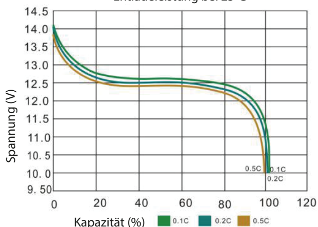
Entladeleistung bei 25°C
