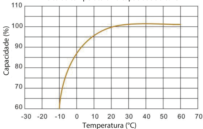
Efeito da temperatura na capacidade a 0.2C
