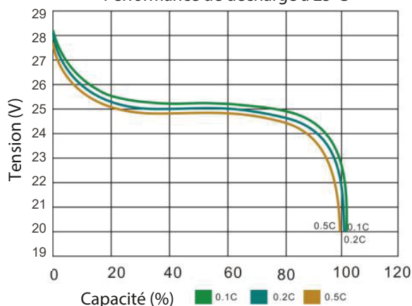
Performance de décharge à 25°C
