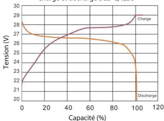
Charge et décharge à 25°C, 0.2C
